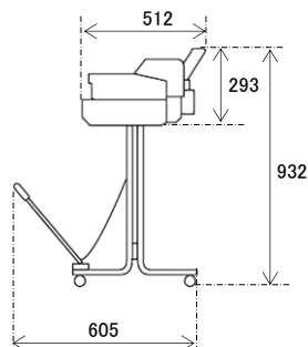
側面 [mm]
