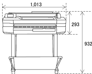
正面 [mm]
