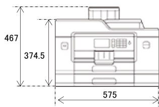
正面 [mm]
