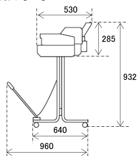
側面 [mm]
