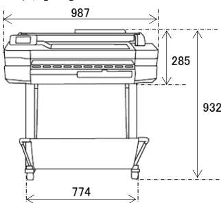
正面 [mm]
